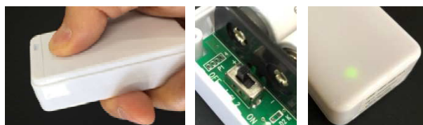
電池交換スライドカバー 電源スイッチ 状態表示LED
